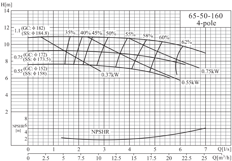
NISO,NIS,NISF 65-50-160/80-50-200
