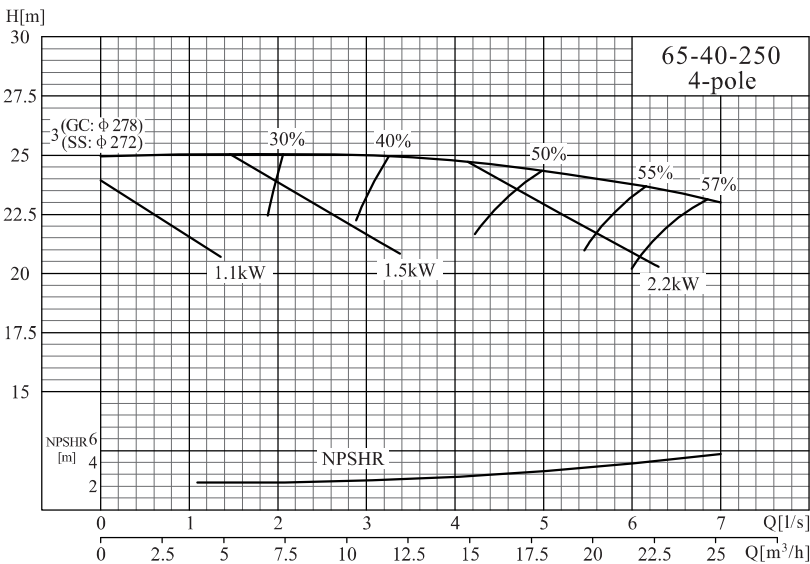
NISO,NIS,NISF 65-40-250/65-40-315
