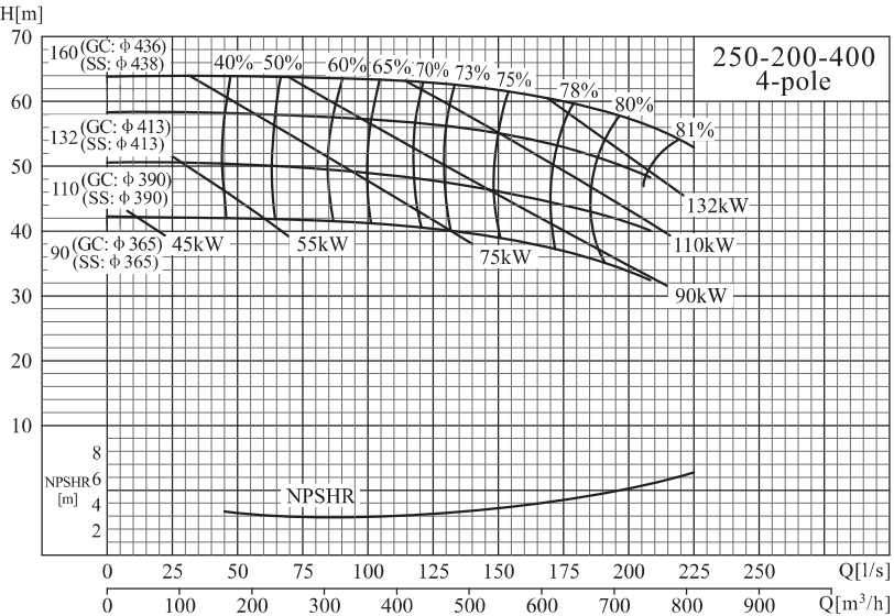
NISO,NIS,NISF 250-200-400/300-250-315(Q)
